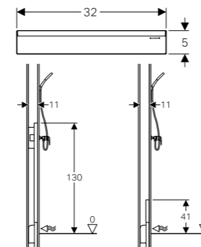
Stenski odtok za prho Geberit
